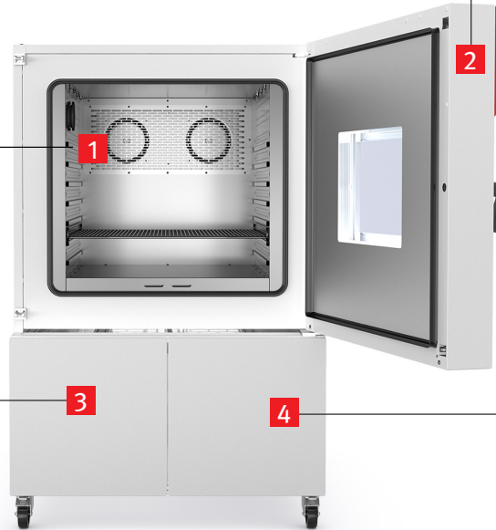
Modell MKF 400
